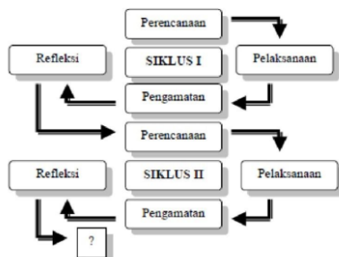
Gambar 1. Siklus PTK
